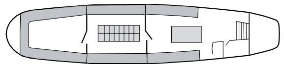
Huvuddäck
